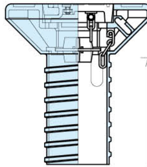
クサリ式
