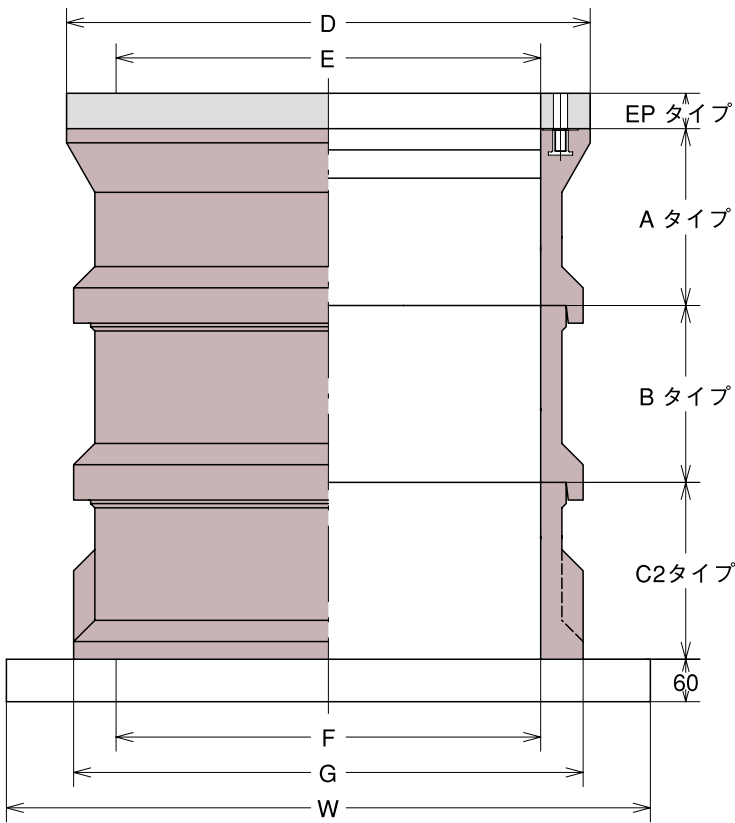
レジソボックス寸法表
